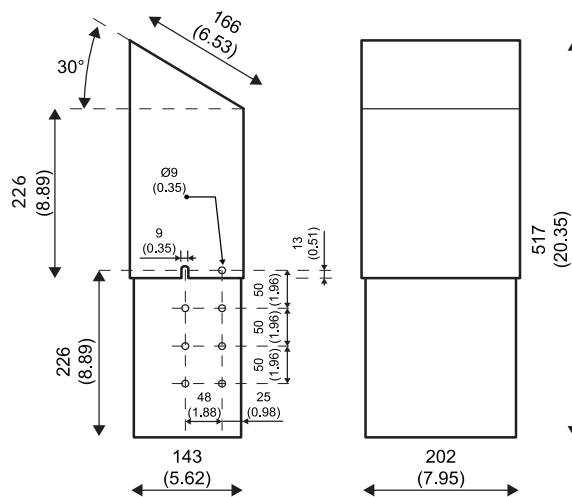
Indoor 90302ZAC
